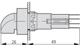
Q...LWK...
