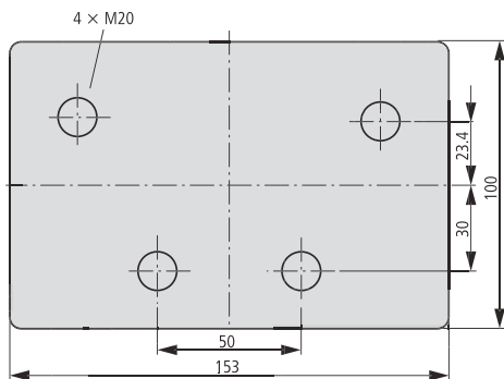
明装外壳 I8
