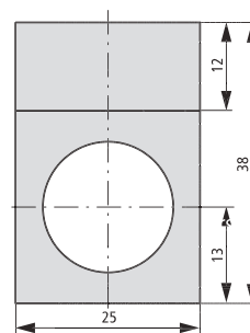
标签安装 Q25TS-...
