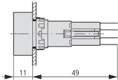
Q25PV... Q25LPV...
