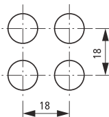
Q18...
