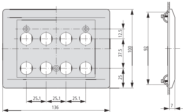
明装外壳 I8
