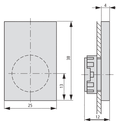
孔塞 Q25AS
