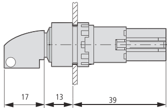
Q...LH-...
