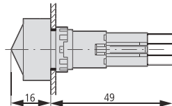
Q...LH-...
