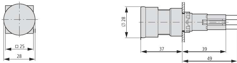
前部固定 Q18, Q25, E89, SRA, VS, M16
