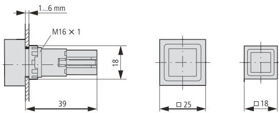
Q...D-... Q...DR-...
